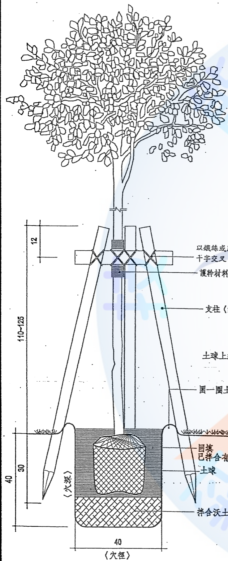
喬木栽植剖面示意圖 S=1/10
