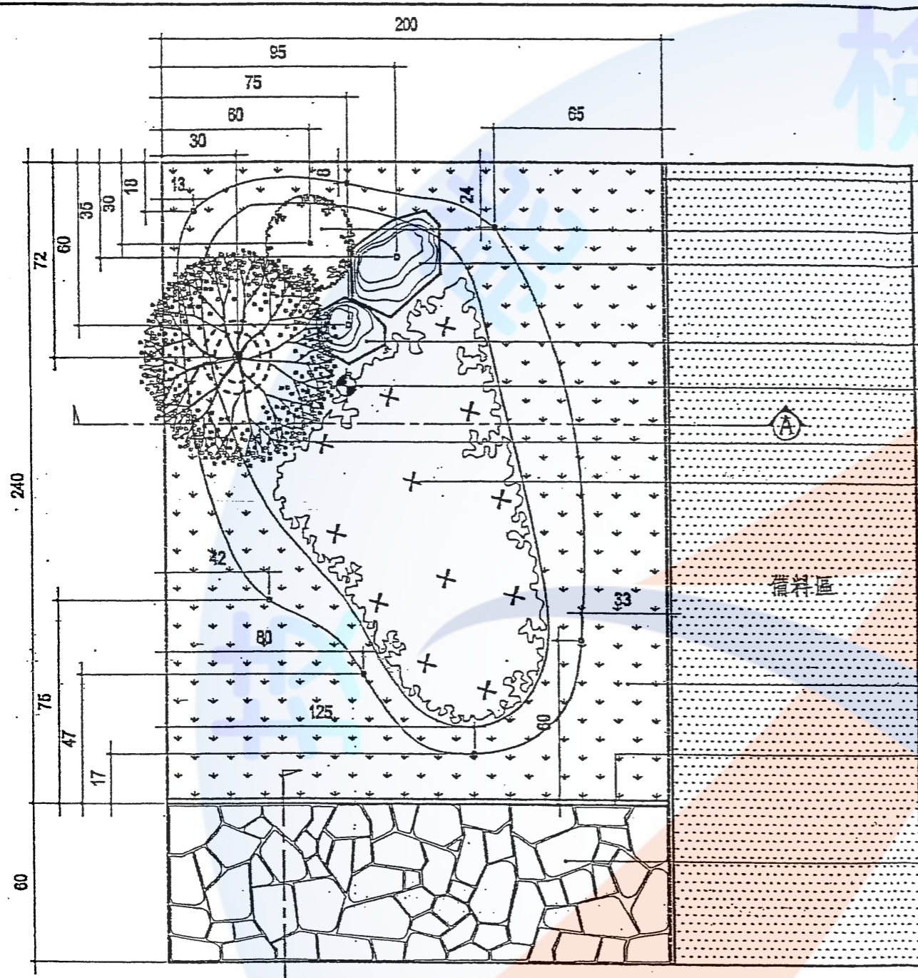
平面圖 S=1/20
