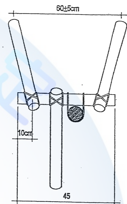
支柱上視示意圖 S=1/10
