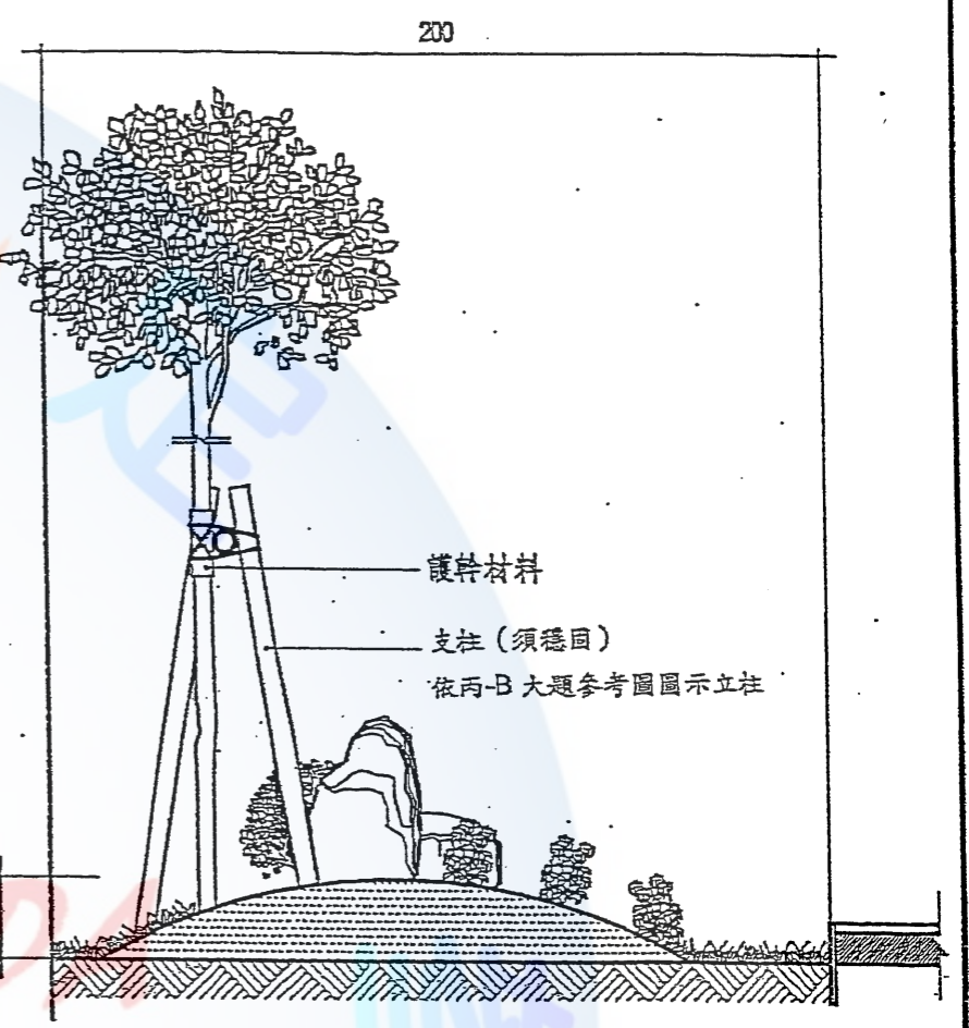
剖面圖 A S=1/20
