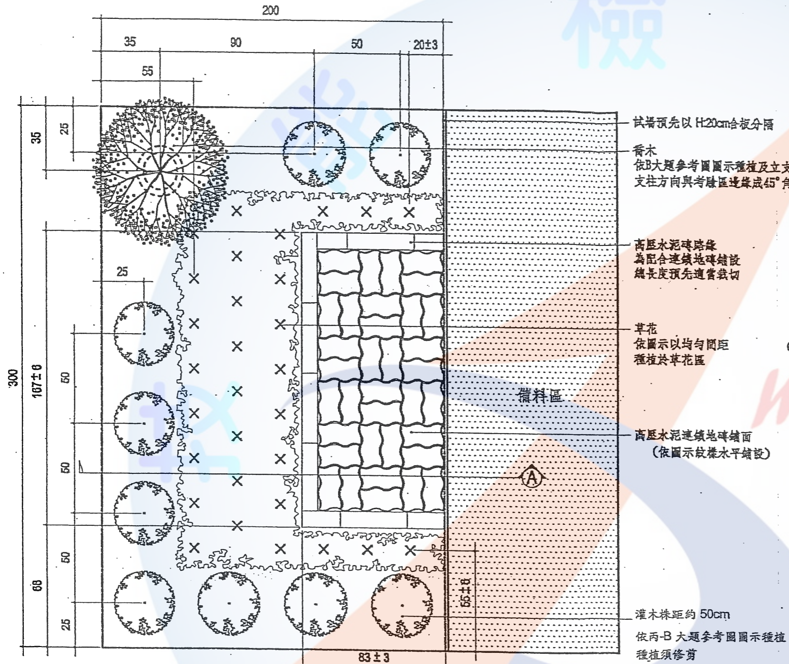
平面圖 S=1/20
