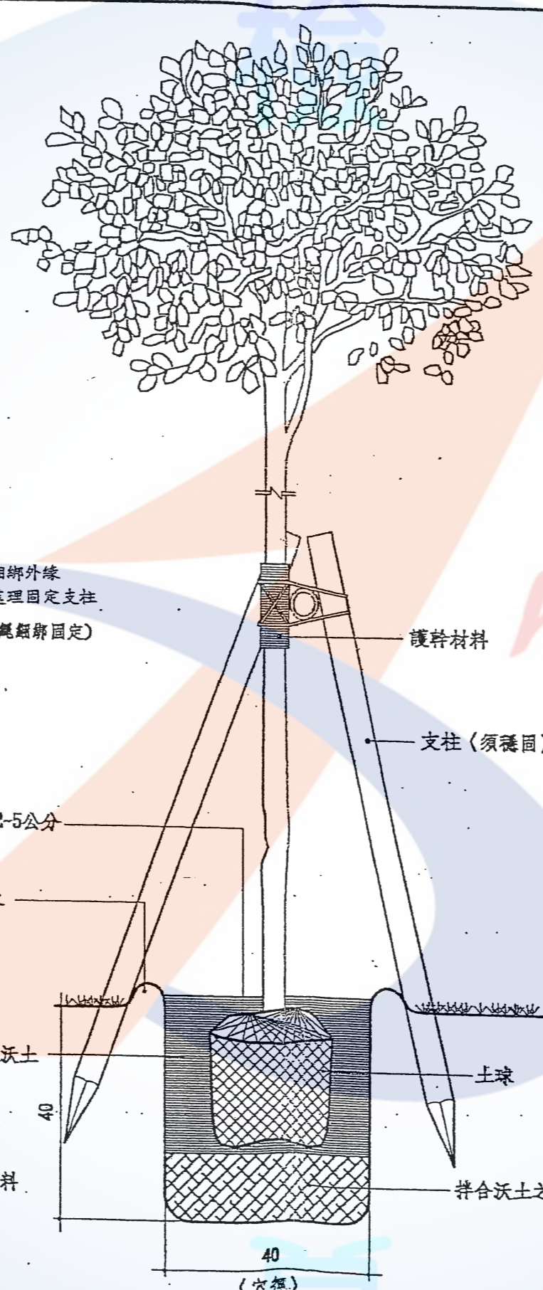
喬木栽植剖面示意圖〈側面〉S=1/10
