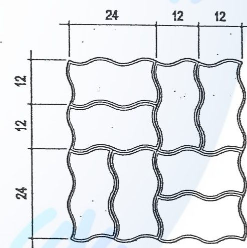
高壓水泥連鎖地磚示意圖 S=1/10
