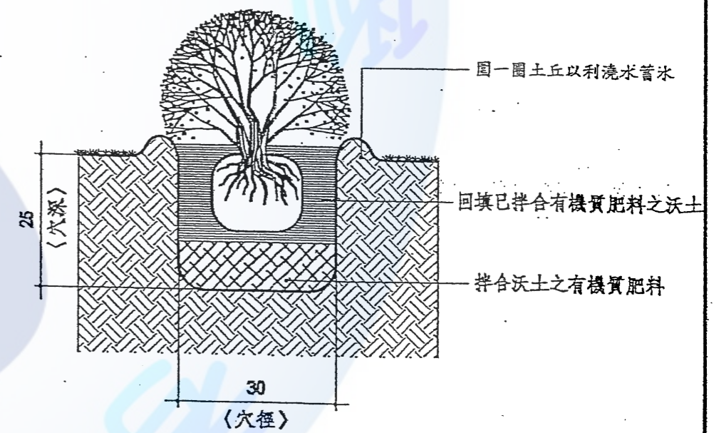
灌木種植剖面示意圖 S=1/10
